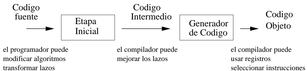
Figura 7.9: Niveles en los que el programador y el compilador pueden mejorar el código
