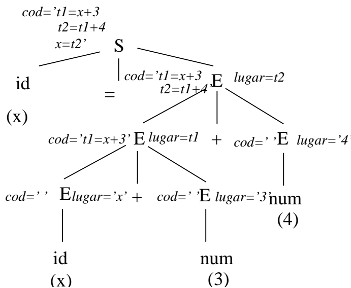
Figura 7.3: Árbol sintáctico para el ejemplo x=x+3+4
