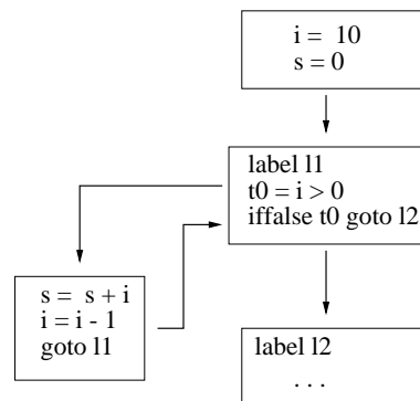
Figura 7.10: Diagrama de flujo
