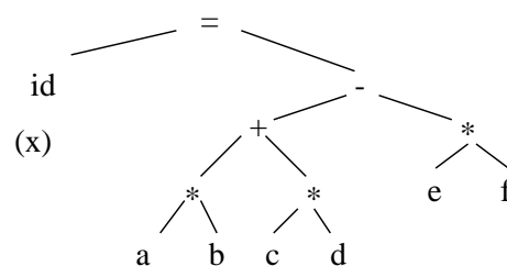
Figura 7.4: Árbol sintáctico para el ejemplo x=a*b+c*d-e*f
