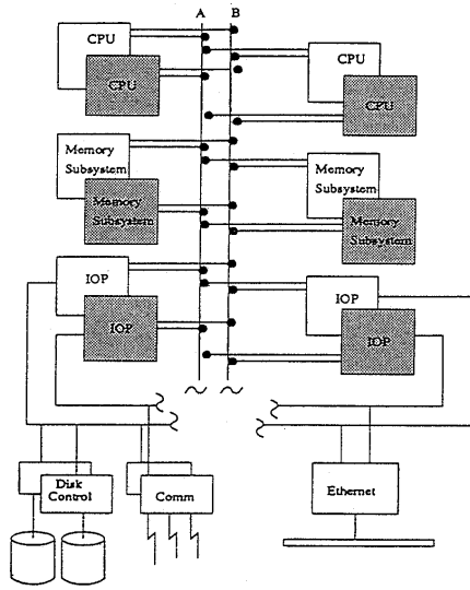
Stratus XA/R Serie 300
